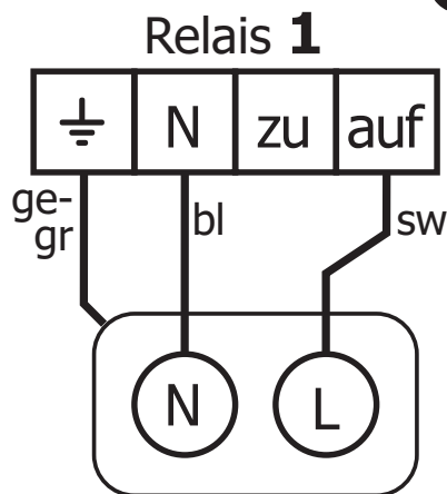
Magnetventil 1 für Rückspülen muß vorhanden sein
