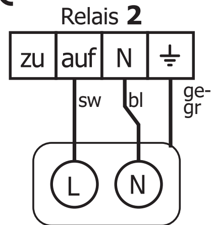
Magnetventil 2 für Klarspülen als Option
